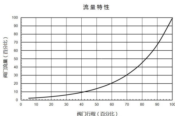
图1 流量特性
