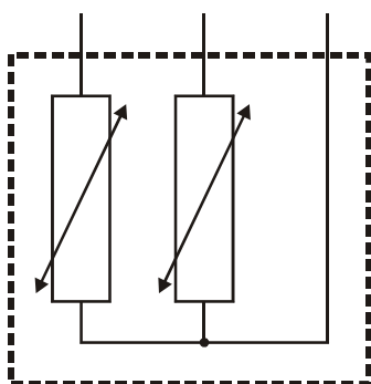
Fig. 4. WPF20 wiring
