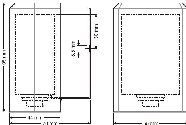
Fig. 1. Dimensions (mm)
